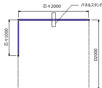
平面図 (角小間)
