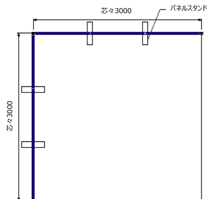
平面図 (角小間)
