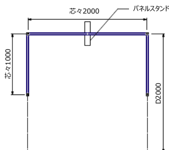
平面図 (中小間)
