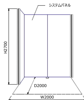
小間姿図 (角小間)
