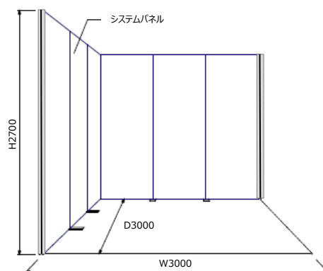
小間姿図 (角小間)
